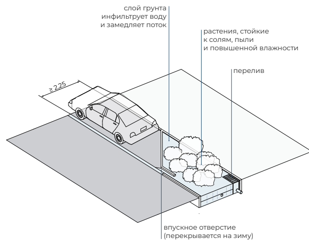
БИОДРЕНАЖНАЯ КАНАВА НА ИСКУССТВЕННЫХ СУЖЕНИЯХ ПРОЕЗЖЕЙ ЧАСТИ
