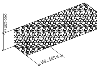
Ограждение территории габионной конструкции
