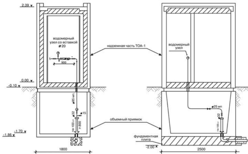
Илл. 5.5.1. ПРИНЦИПАЛЬНАЯ СХЕМА МОНТАЖА ОБЩЕСТВЕННОГО ТУАЛЕТА, ЦЕНТРАЛИЗОВАННОГО ПОДКЛЮЧЕНИЯ
